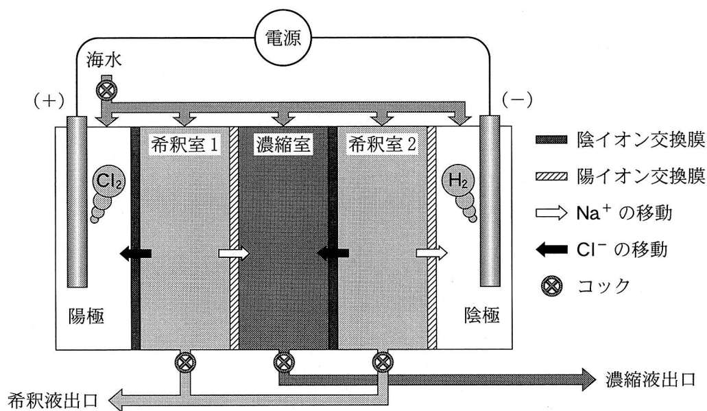
図 2 イオン交換膜法による海水の濃縮装置の模式図
