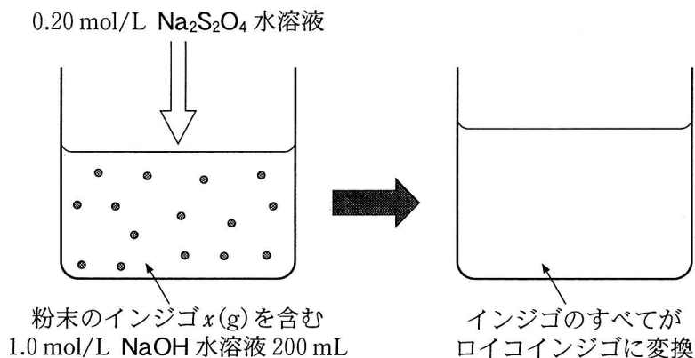
図2 インジゴをロイコインジゴに変換して水に溶解させる実験
