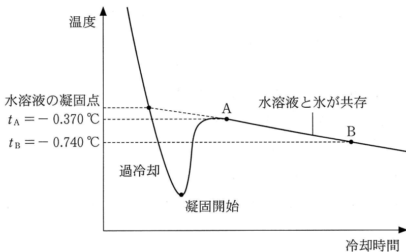
図3 シヨ糖水溶液の冷却曲線
