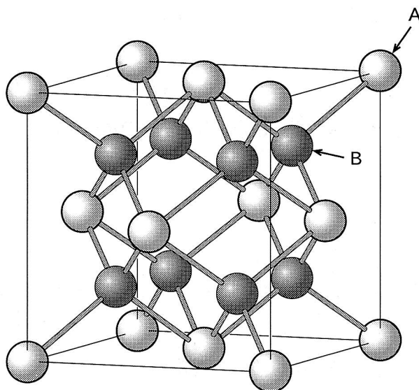
図1 陽イオンAと陰イオンBからなる、ある結晶の単位格子
