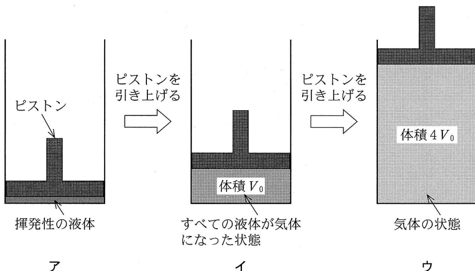
図 2 揮発性の純物質の液体のみを入れた密閉容器のピストンを引き上げたときの模式図
