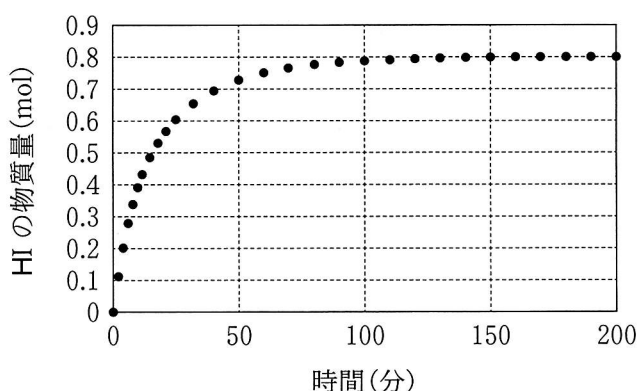
図 1 HI の物質量の時間変化
