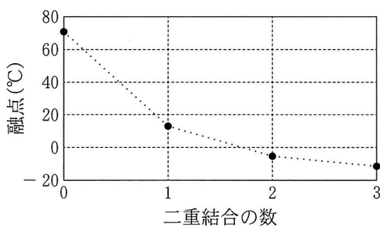
図 4 炭素数 18 の脂肪酸における炭化水素基中の二重結合の数と融点の関係
