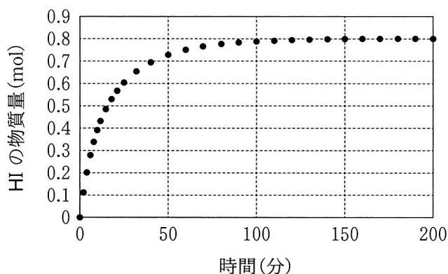
図 1 \text{HI} の物質量の時間変化
