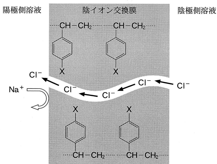
図 3 \text{Cl}^- の陰イオン交換膜透過の模式図
