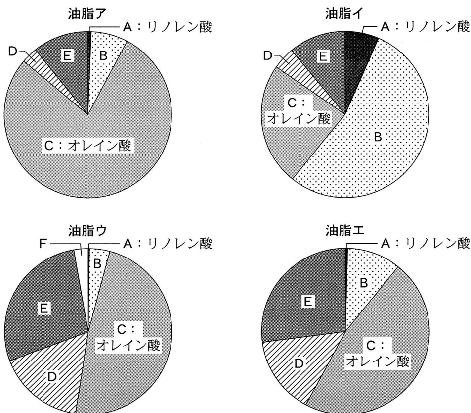
図5 油脂ア～エを加水分解して得られる脂肪酸A～Fの含有率(質量パーセント)
